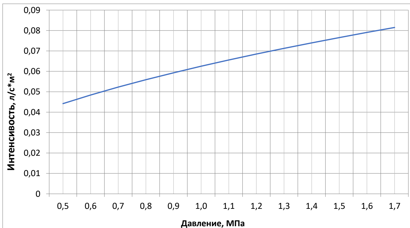
График зависимости интенсивности орошения от давления на площади 16 м², защищаемой одним оросителем с высоты 2,5 м
